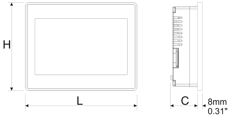
Fig. 4: Dimensions – TX707(HB)
