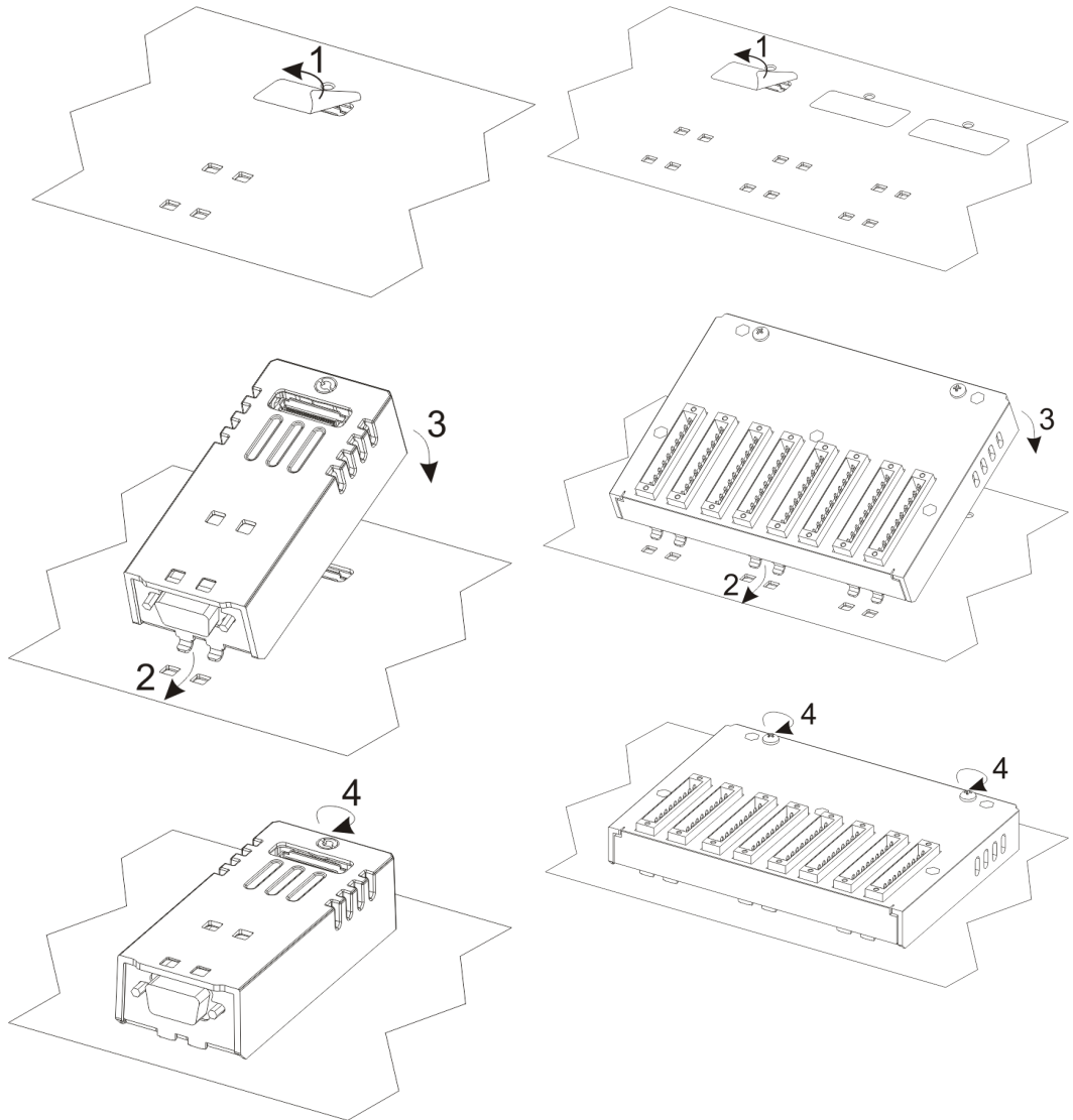
Fig. 8: Installing plug-in modules (e. g. TX-CAN, TX-IO-DX06)
