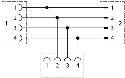
电路图
