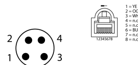
Schéma zapojení
