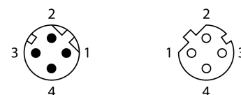
Schéma zapojení
