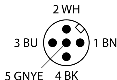
Schéma zapojení
