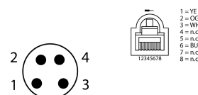
Schaltplan
