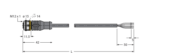
Maßbild Typ Ident-No.
