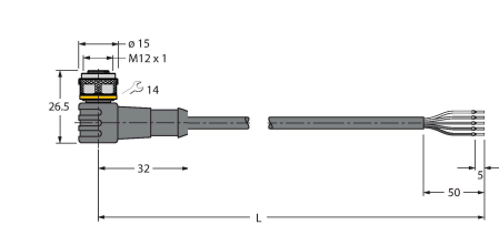
Maßbild Typ Ident-No.
