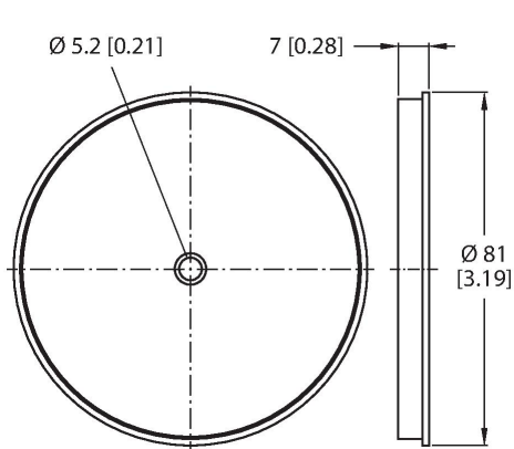
Dibujo acotado Tipo N.º de ID
