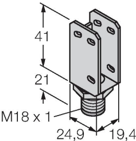
Dibujo acotado Tipo N.º de ID RKC4.4T-2/TEL 6625013
