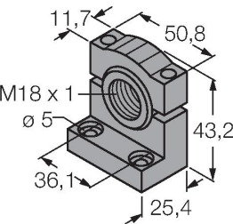
SMBQS18A 3069721 escudra de montaje, acero inoxidable, para rosca de 18 mm
