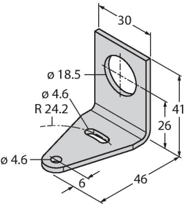
SMBQS18A 3069721 escudra de montaje, acero inoxidable, para rosca de 18 mm
