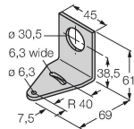
SMB30A3032723 Ángulo de montaje, en ángulo recto, acero inoxidable, para sensores con rosca de 30 mm
