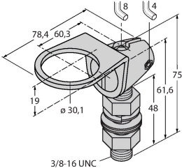
SMB30FA3074005 Montagewinkel; Werkstoff VA 1.4401
