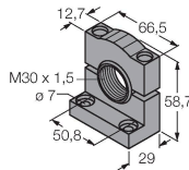
SMB30SC3052521 Soporte de montaje, PBT negro, para sensores con rosca de 30mm, orientable
