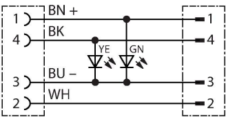
diagrama de conexiones
