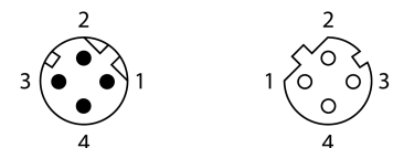
schakelplan
