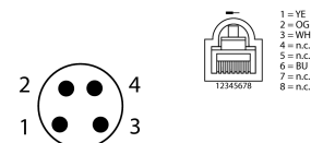
schakelplan
