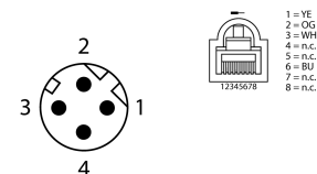
schakelplan
