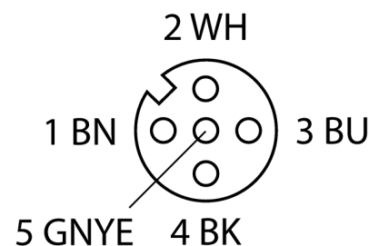
schakelplan
