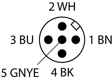
schakelplan
