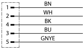
schakelplan
