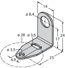
Uchwyt montażowy, VA 1.4401, dla serii T8 lub T8L
