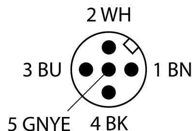
Schema de conexiuni
