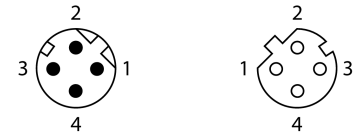
Devre şeması
