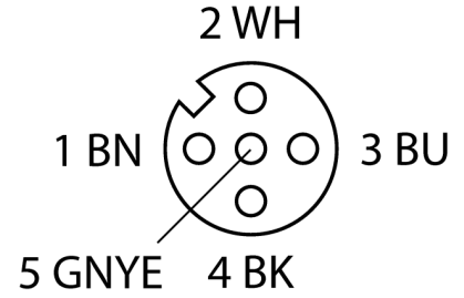
Devre şeması
