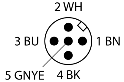
Devre şeması
